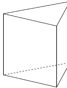
[三角柱]
