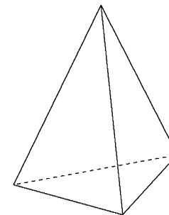
[三角錐]
