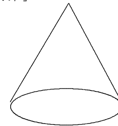
[円錐]
