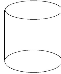
[円柱]
